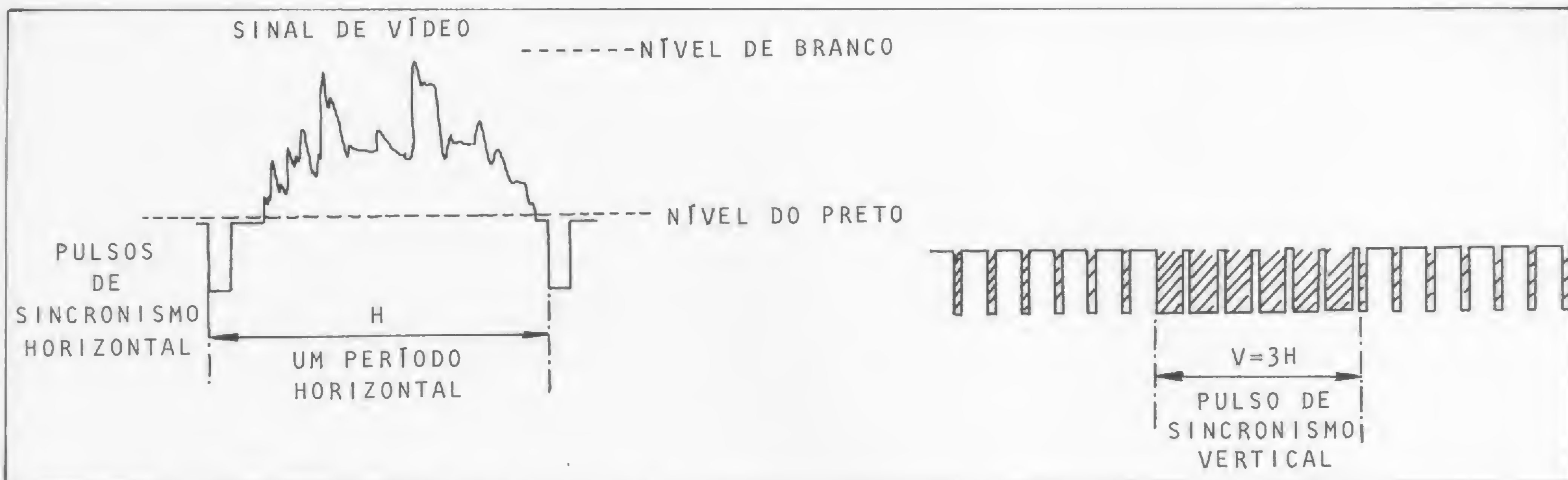
Figura 2 — Apresentação dos pulsos de sincronismo.
